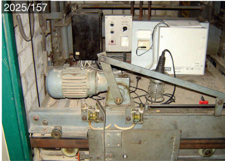
OSMA Typ 1 telescope
