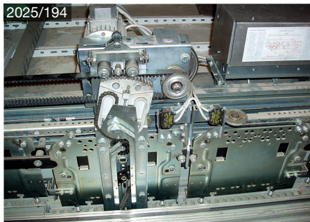
Prisma Linear DOS center
