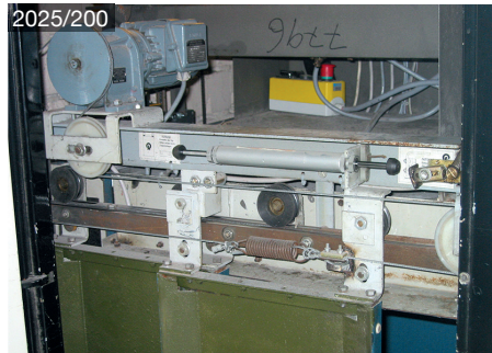
Rathgeber Drahtseil telescope
