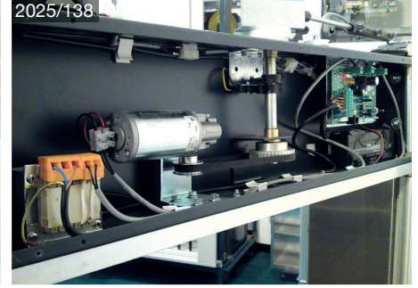
METRON Folding door
