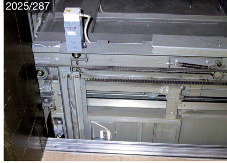
Thyssen M2T W1, G1, D1 telescope
