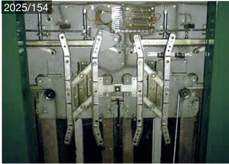
ORONA center
