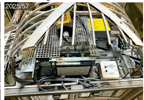
GILGEN folding door
