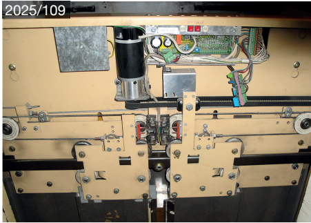
Kone Isola center
