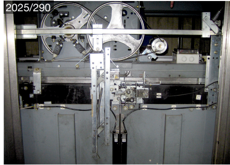
Thyssen M2Z D6 center
