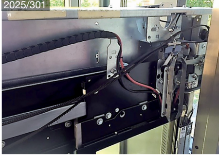
Thyssen VF400 telescope
